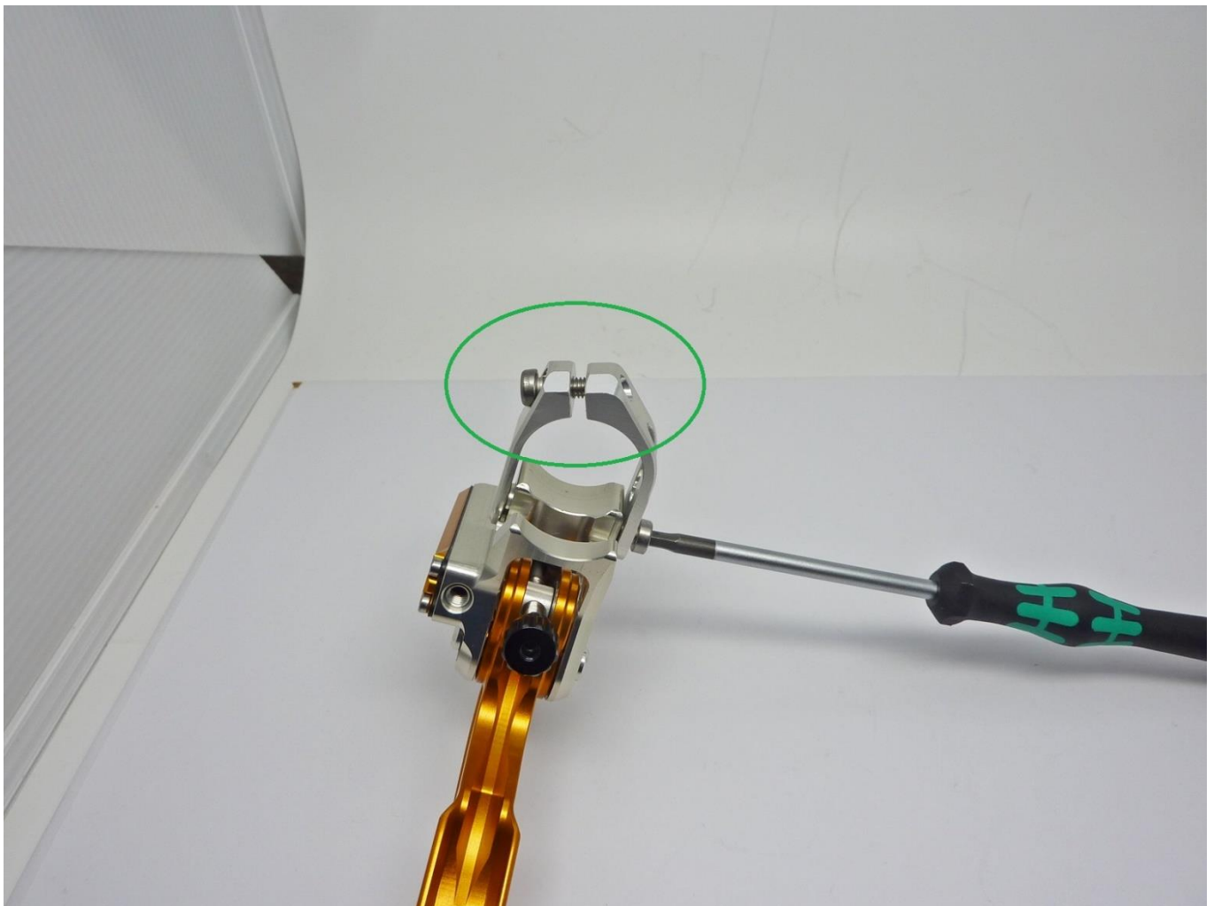
Abb. 5: Frässhelle an DRT Pumpe mit Schrauben angesetzt
